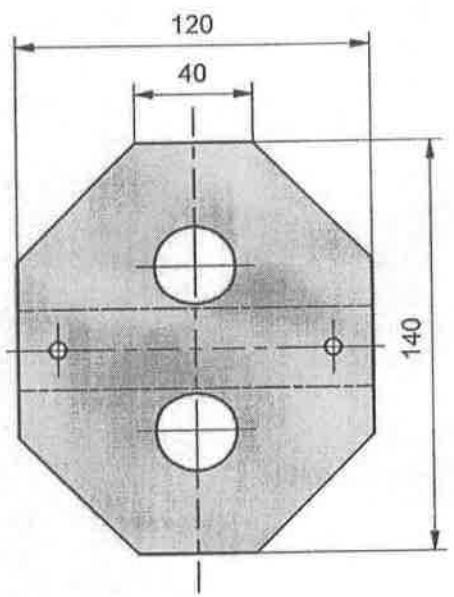
RAZVIJENI OBLIK R1:2,5
